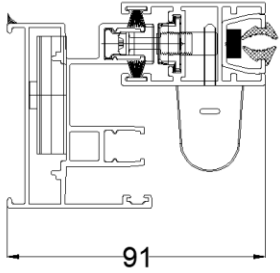
JAMB VISIBLE WIDTH
