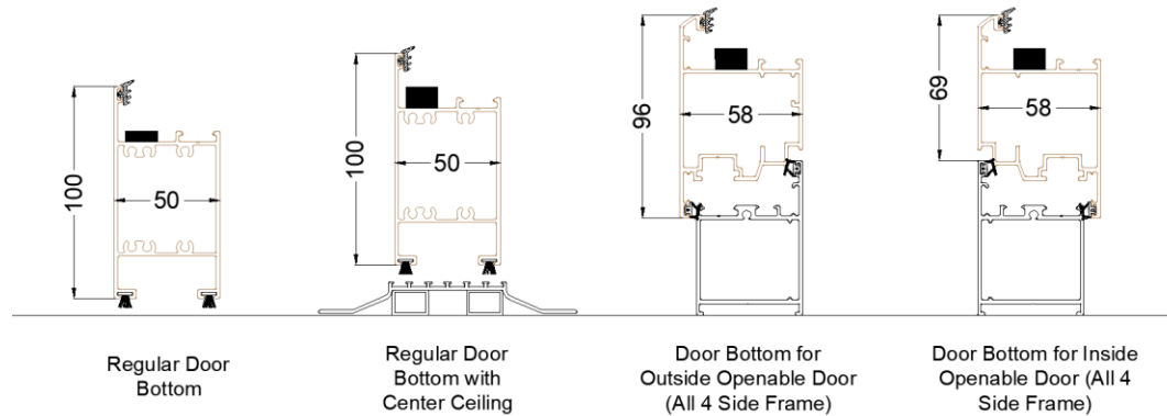
DOOR BOTTOM POSSIBLE COMBINATION
