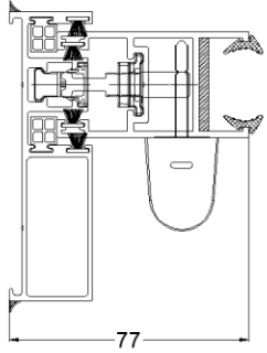
JAMB VISIBLE WIDTH
