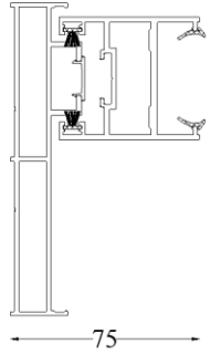
JAMB VISIBLE WIDTH
